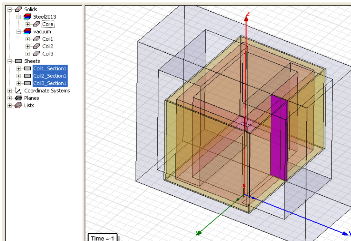
Рисунок 4 – Конечный вид сечений.
