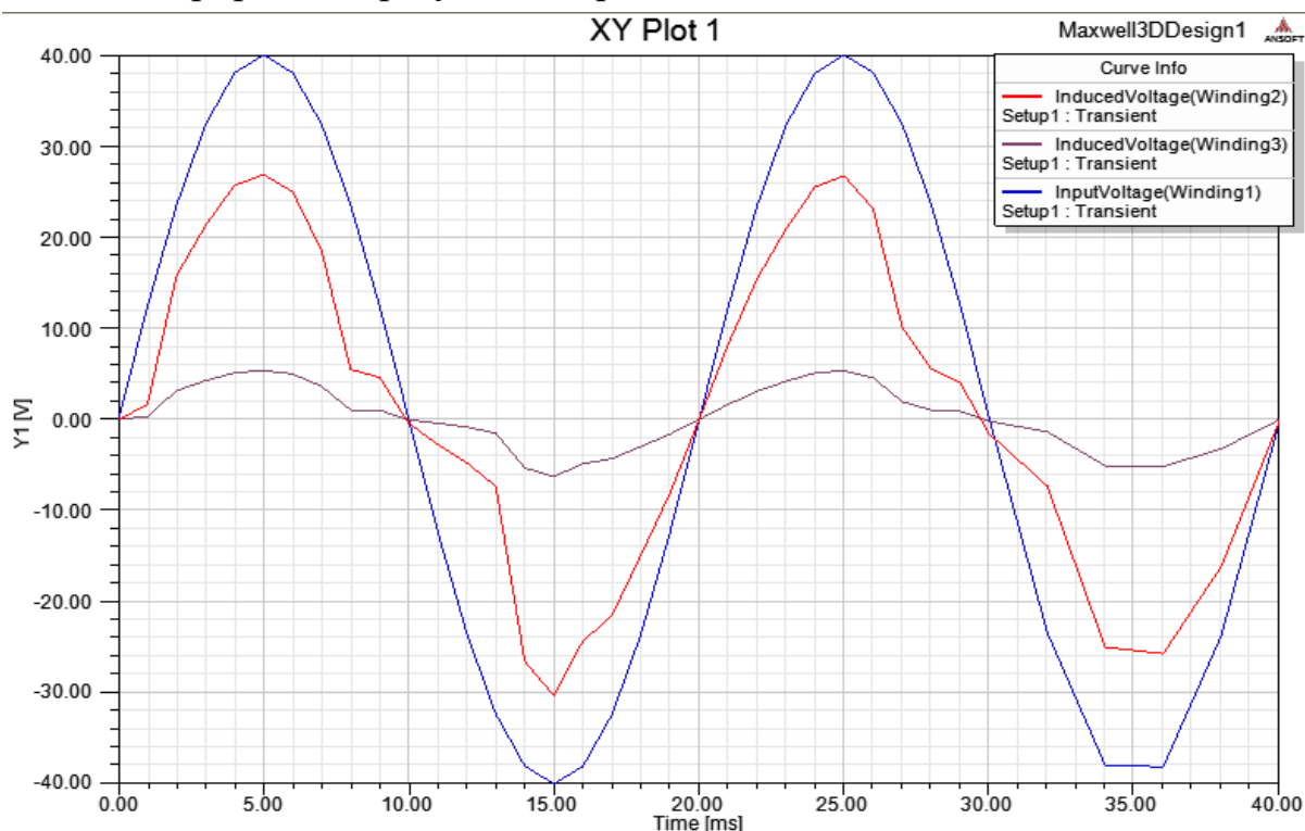
Рисунок 6 – графики входного и индуцированного напряжения.
