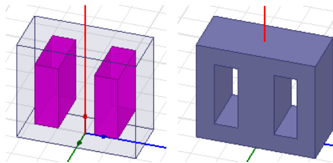
Рисунок 2 – Построение геометрии сердечника.
