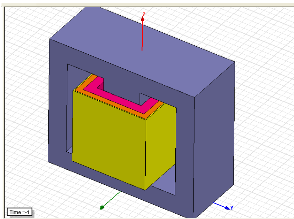
Рисунок 3 – Построение геометрии обмоток.
